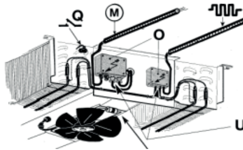
Fig. 4 BMD... - SMD...
