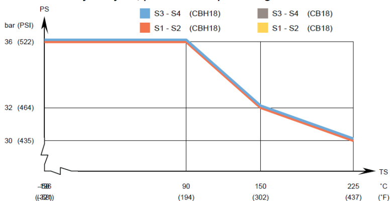
CBH18 – PED-hyväksyntä, paine- tai lämpötiladiagrammi
